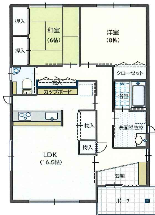
1階平面図
